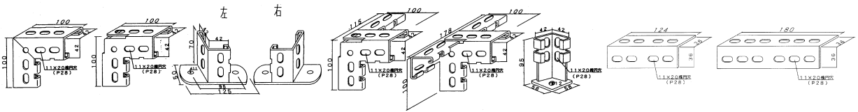
ジョイント金具-1 コーナー ジョイント金具-2 通しコーナー ジョイント金具-3 左・右ストッパー ジョイント金具-4 三方通しコーナー ジョイント金具-5 四方通しコーナー ジョイント金具-6 台座 ジョイント金具-7 アングル連結金具 ジョイント金具-8 アングル連結金具
