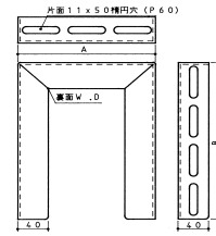
【M-S タイプ】 片面穴明
