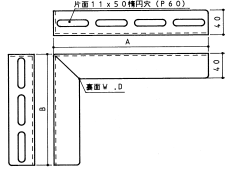
【L-S タイプ】 片面穴明
