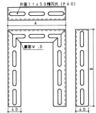
【M-W タイプ】 両面穴明
