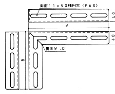
【L-W タイプ】 両面穴明
