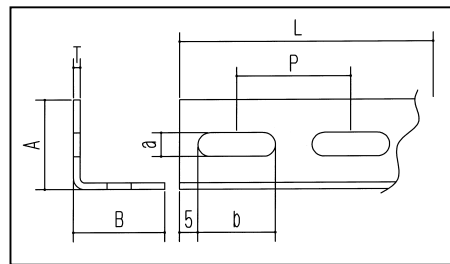
寸法図
