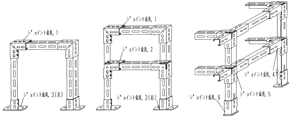
ジョイント金具-1 コーナー ジョイント金具-2 通しコーナー ジョイント金具-3 左・右ストッパー ジョイント金具-4 三方通しコーナー ジョイント金具-5 四方通しコーナー ジョイント金具-6 台座 ジョイント金具-7 アングル連結金具 ジョイント金具-8 アングル連結金具
