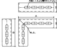
【L-W タイプ】 両面穴明(150・210)
