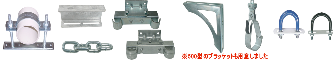
配-51～55Uﾊﾞﾝﾄﾞ防振Uﾊﾞﾝﾄﾞ 配-566 ﾎｲﾄﾞ管止金具 配管固定ﾊﾞﾝﾄﾞ
