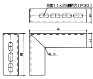
【L-S タイプ】 片面穴明(150・210)
